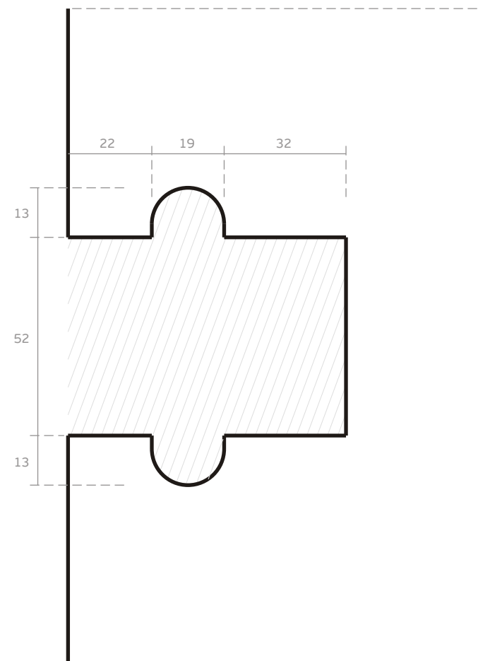
GC35 - Entalhe no vidro / Glass cut / Taladro en el cristal
