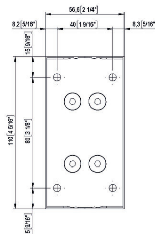
Vista frontal 2
