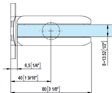
Sección transversal 1
